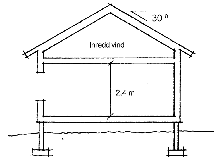
Sektion
