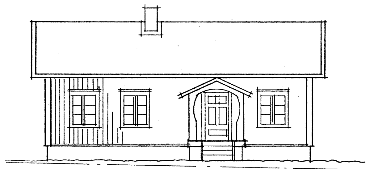
Fasad söder
