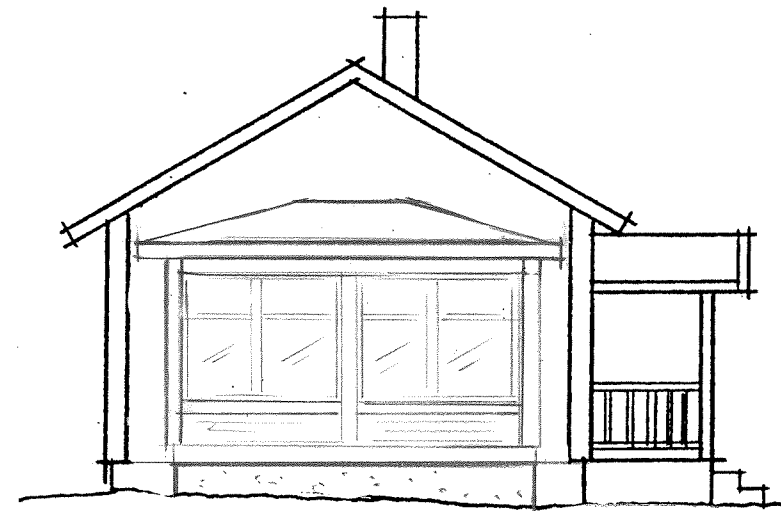
Fasad väster
